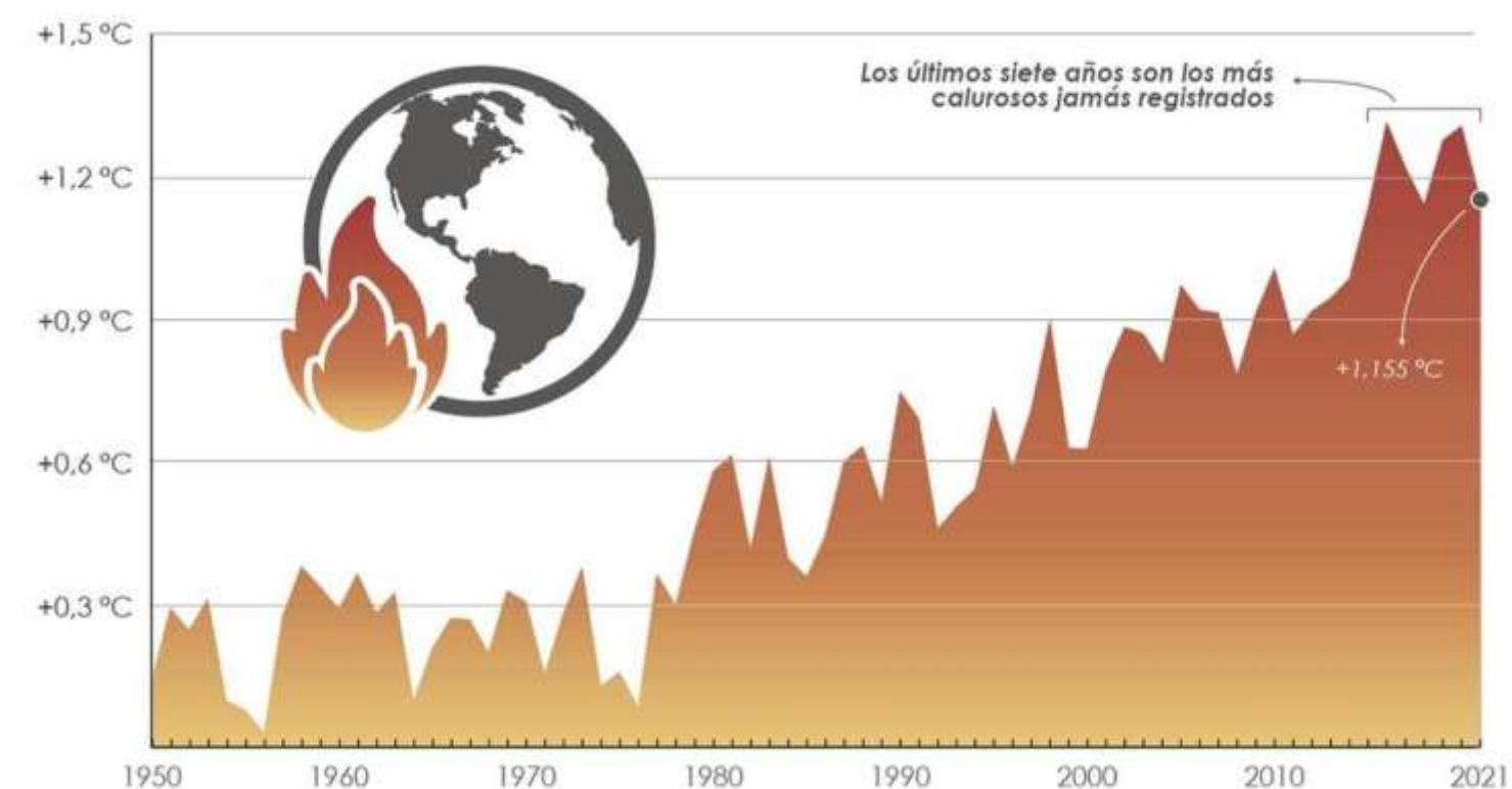
Cambio en la temperatura media global anual con respecto al periodo 1850-1900
